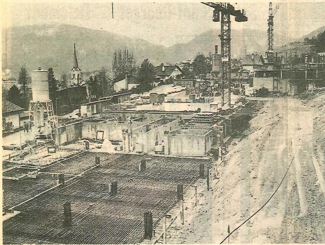
Vue générale du chantier.
